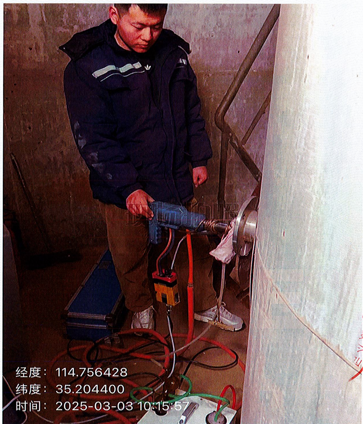
图 2-1 有组织检测 3#焚烧废气排放口 DA003
